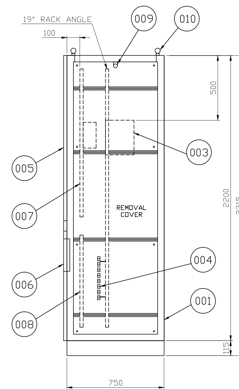
R.H. SIDE VIEW
