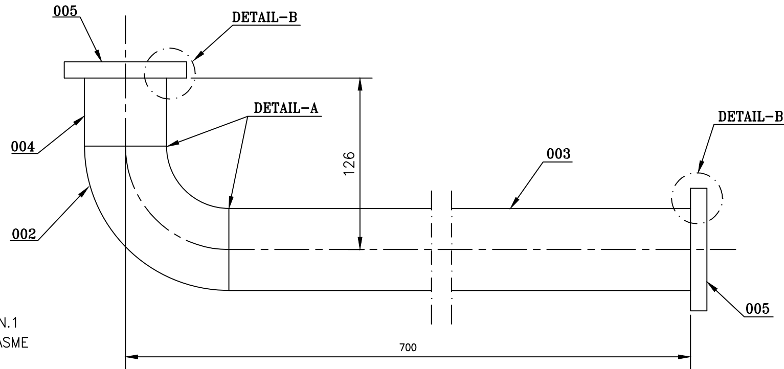
ASSLY.OF ITEM 001,VAR.00
