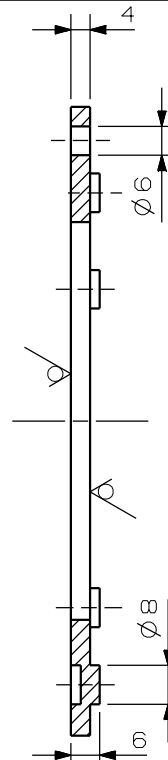
SECTION A-B
